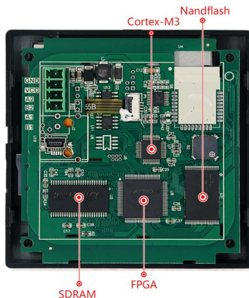
1-1 硬件配置图
